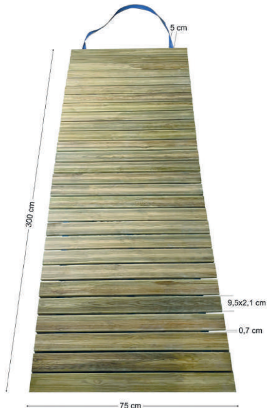
Lane / E2200 Διάδρομος παραλίας εμποτισμού pine / 300x75 Πάχος ξύλου 21mm / Σύνδεση με ιμάντες προτυλενίου
